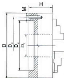
на планшайбу тип 3504 DIN 6350
