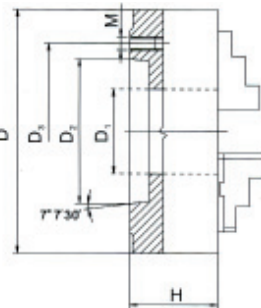
на конус тип 3534 DIN 55027
