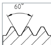
ВСТАВКИ МЕТРИЧНІ 60°
