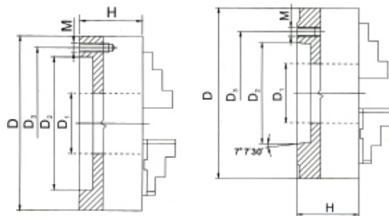
на планшайбу тип 3504 DIN 6350
